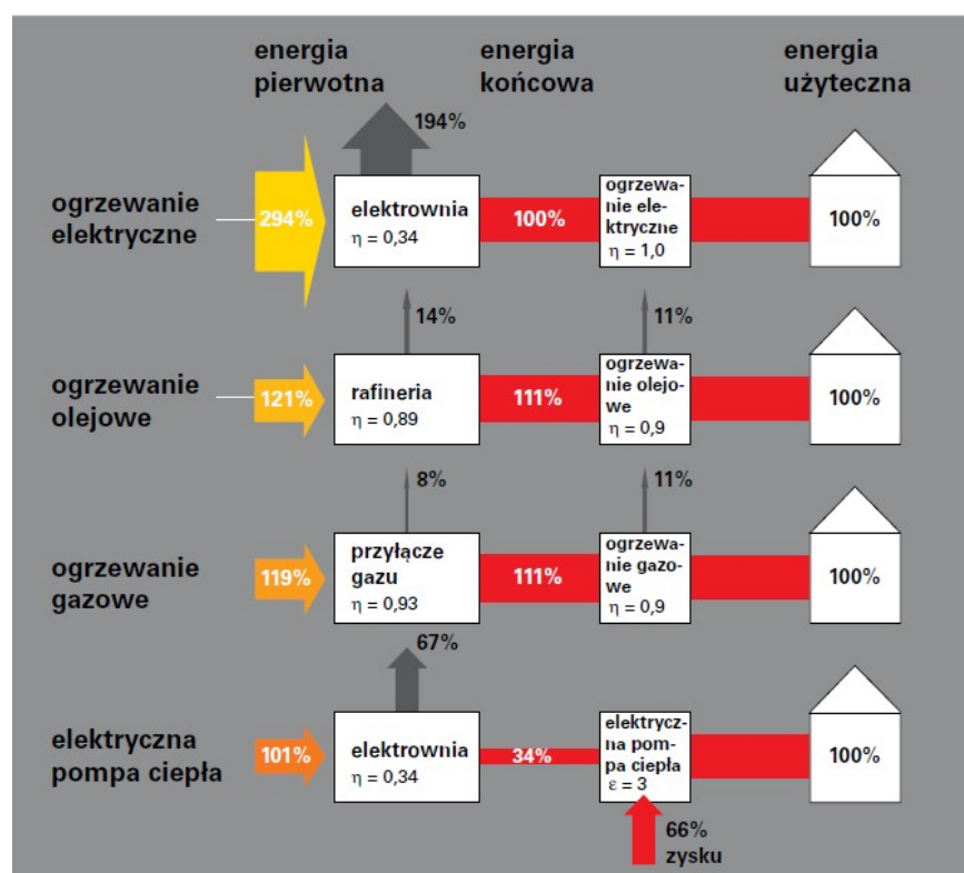
Rys.21. Łańcuch przekształceń energii z uwzględnieniem pompy ciepła Źródło: https://portpc.pl
